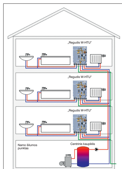
Sistemos schema
